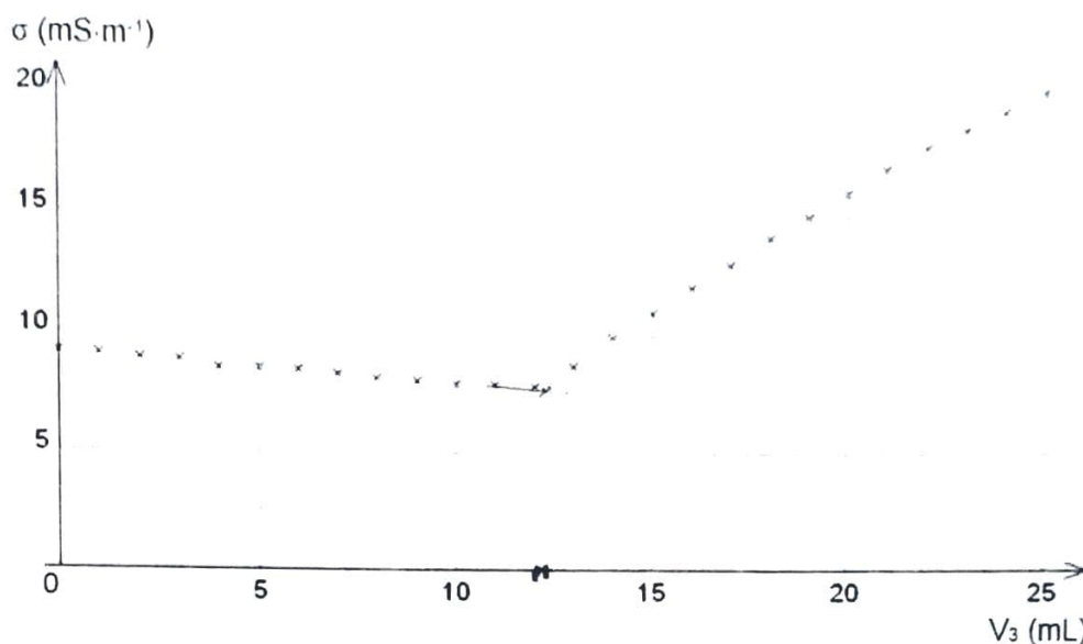
figure 2 : évolution de la conductivité \sigma du mélange dans le bécher en fonction du volume V_3 de solution de nitrate d'argent versé
