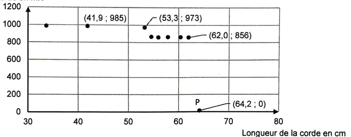
Figure 2. Représentation graphique de la valeur de la tension de la corde en fonction de sa longueur
