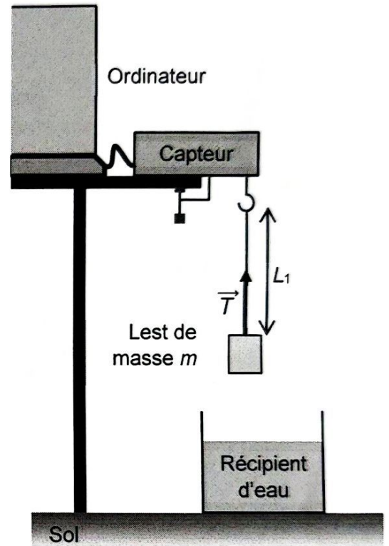
Figure 1. Schéma du dispositif expérimental
