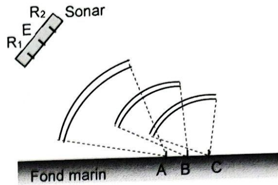
Figure 4. Propagation des échos vers le sonar
