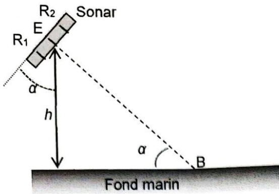
Figure 3. Géométrie du dispositif
