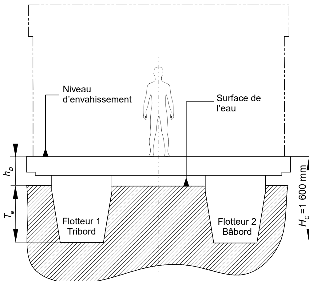
Figure 2 : vue en coupe du Boathome.
